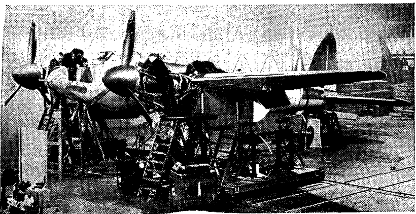
Britaniyan texlîtek balafr hene jê re dibêjin « mûskitos »; balafrne hûr û sivik, balafrine keşif û nêçirvaniyê. Ev in çend « mûskitos ». Mihendis û emele di hola Fabrikê de perçeyên wan li hev siwar dikin.
