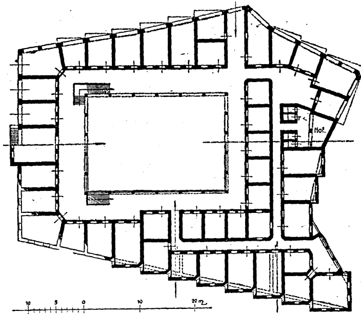
وینه ۴۵: کاروانسه‌رای حه‌سه‌ن پاشا
