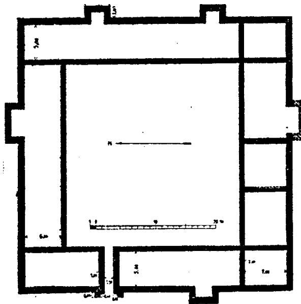
وینہ ۲: زہردہ خان لہ تہفتہق لہ لایہن (E. Rauschenberger) وہ نہخشہکھی وەرگیراوه (Expedition 1913. Freiherr von Oppenheim)
