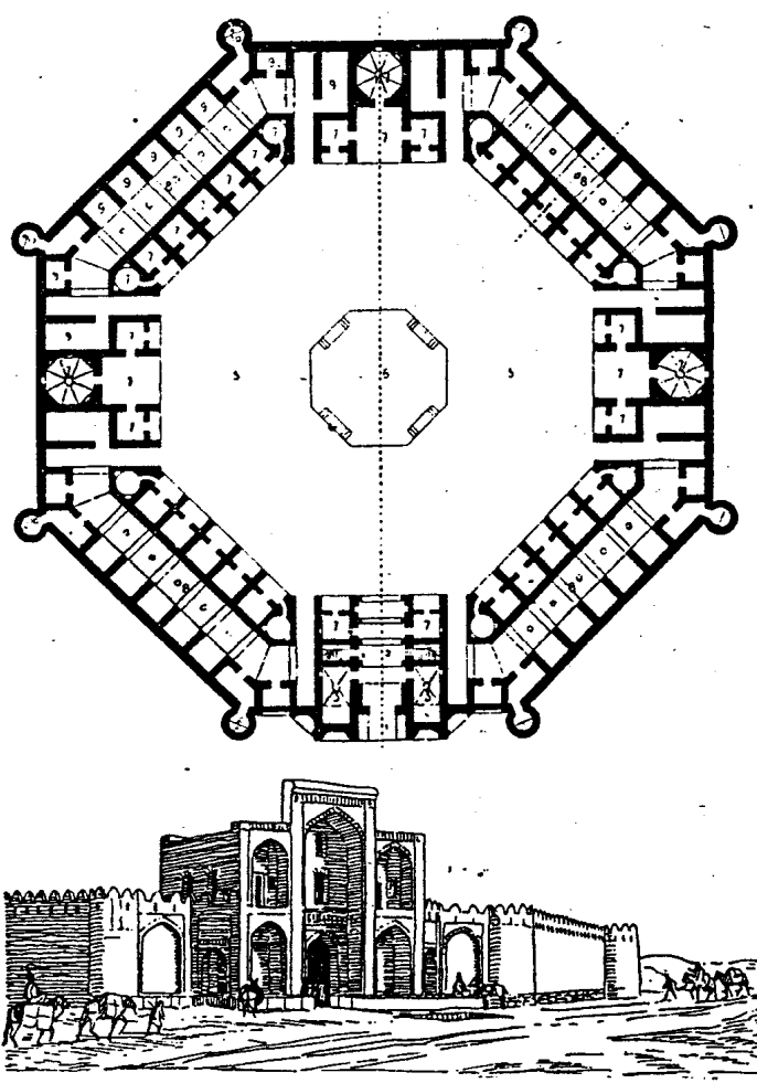
وینه ۲۴: کاروانسرای نهمین آباد لسه‌ر ریگای نسه‌فه‌هان به‌ره‌و شیراز له (P. Coste, Monuments modernes des la perse) وەرگیراوه.
