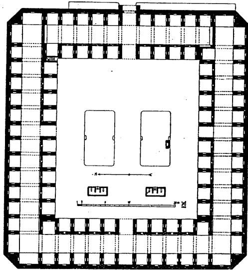
وینہ ۸: خانی مه‌حاویل له‌سه‌ر جاده‌ی به‌غدا- که‌ر به‌لا (نه‌خشه‌ی ناسوویی)
