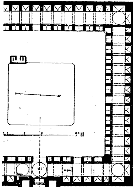
وینه‌ی ۶: نه‌خشه‌ی ئاسۆیی خانی ناسری‌یه له‌سه‌ر جاده‌ی به‌غدا- حله
