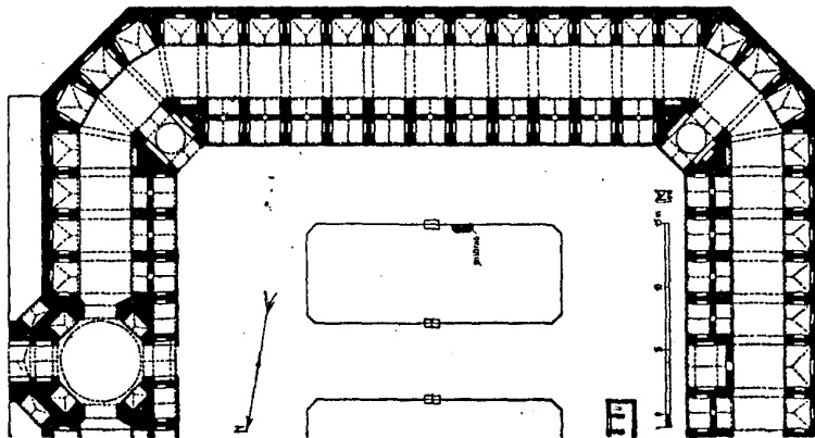
وینه ی ۱۸: خانی حه سوه له سهر جاده ی به غدا- حله
