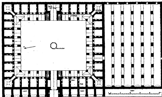
وینەیی ۳۵: نەخشەیی ئاسۆیی کاروانسەرایی دەلال لە شاری ئامەد (دیاربەکر)
