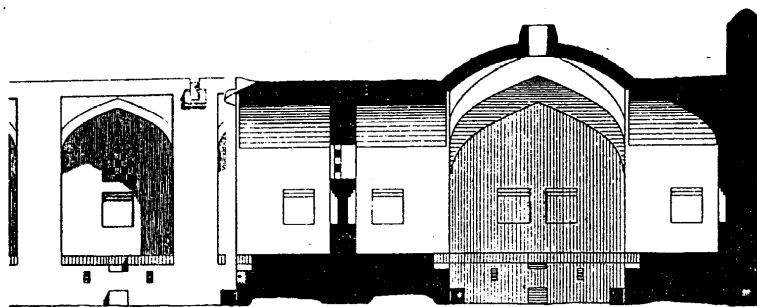
وينە ۶۰: ديمەن و برگەى كاروانسەراييك. برگەكە كونجەكانى
