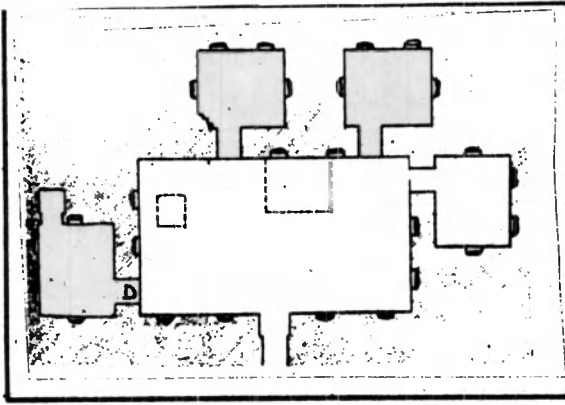
Urartu kralı I. Argiştı'nın Van kayalığındaki mezarının planı
