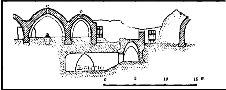
شێوهی ٣٣- نیوه رو (پهروڤیل) ی خانووی تک له گوندی مهراغه
