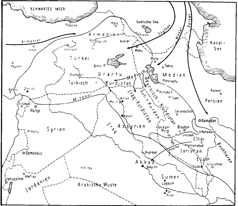
Übersichtsskizze 2: Die sprachliche Indogermanisierung von Ostasien, Kurdistan und Iran im 1. Jt. v. Chr.
