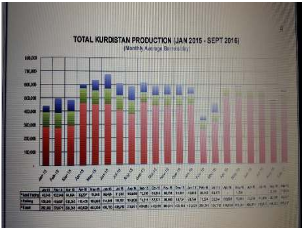
نەخشەى كۆى بىرى بەرهمى نەوتى هەرىمى كوردستان لە مانگى ٢٠١٥/١ تا مانگى ٢٠١٦/٩
