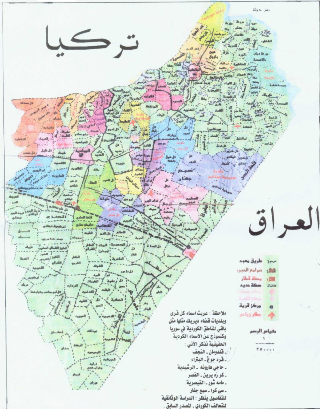
خريطة توضح قرى وبلديات قضاء ديريك (المالكية) حالياً.
