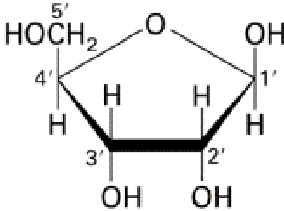
Ribose
