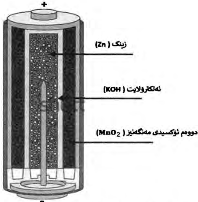
وتتەى ۲ - ۳: پىكھاتەى پاترى سەرەتائى ئەلكالى
