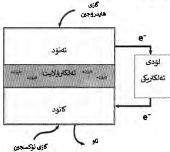
ويئەى ۱ - ۷: پىكھاتەى خانەى سووتەمەنى
