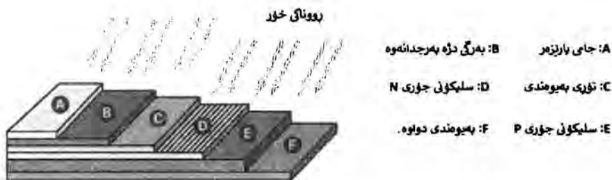
ويته ي ۵ - ۱۲ : پيگهاته سهره كيه كانى خانه ي خورى
