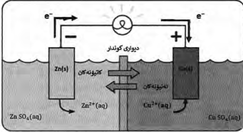
ويتى ۱ - ۱۵: خانەى گەلفانىكى مس - زىنك
