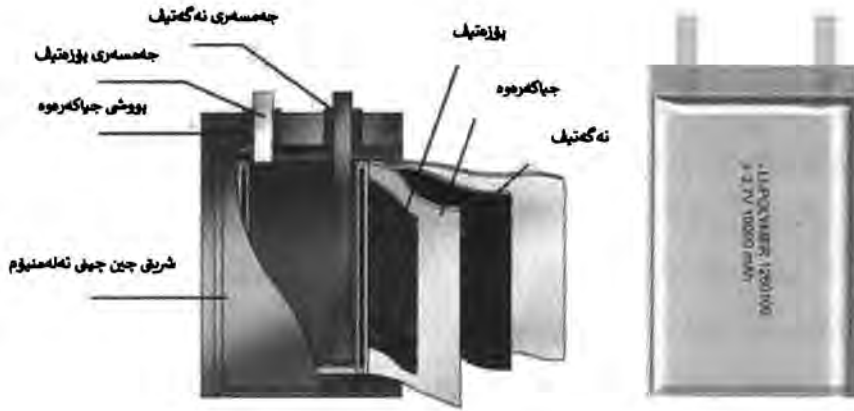
۴ - ۲۷ : پىكھاتەى پاترى لىتىيۇم-پۆلىمەر
