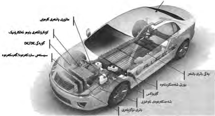
۵ - ۴ : پىكھاتە سەرەككەكانى ئۆتۈمبىلى كارەبى
