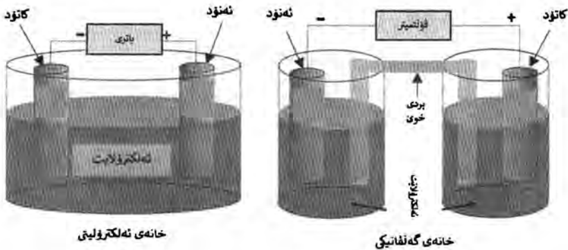
۱ - ۱۴: جياۋازى خانەى ئەلكترولىتى لەگەل خانەى گەلقانىكى
