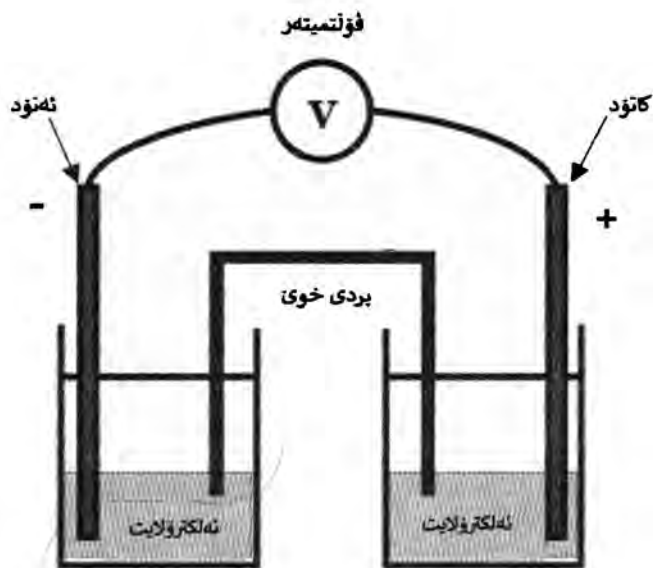
۱ - ۵: پېكھاتەى خانەى گەلفانى
