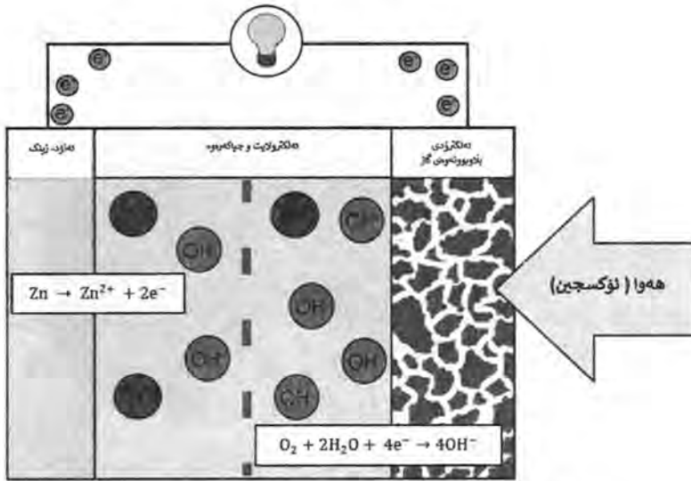
وینته ۲ - ۴ : کارلیکه کانی نیو پاتری زینک-هوا
