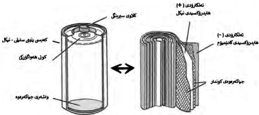
وینه ی ۴ - ۲۲ : پیکهاته ی پاتری نیکل-کادیمیۆم
