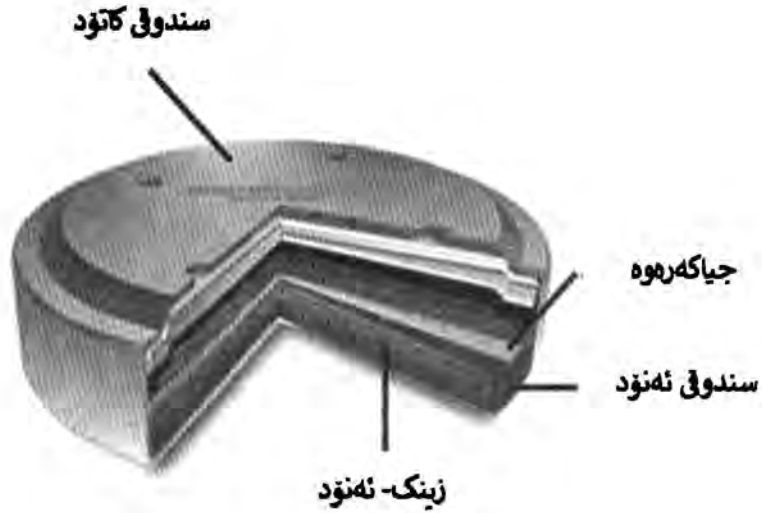
ۋىتەى ۳ - ۳ : پىكھاتەى پاترى زىنك-ھەۋا
