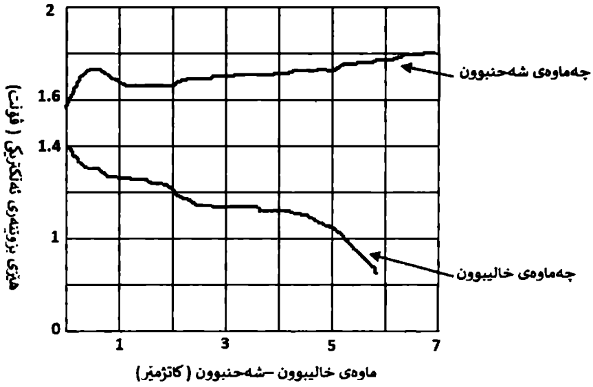
۴ - ۲۱ : چەماوھى خالىبوون-شەخنىبوونى خانەى پاترى نىكل-ئاسن ( پاترى ئەدىسۇن)
