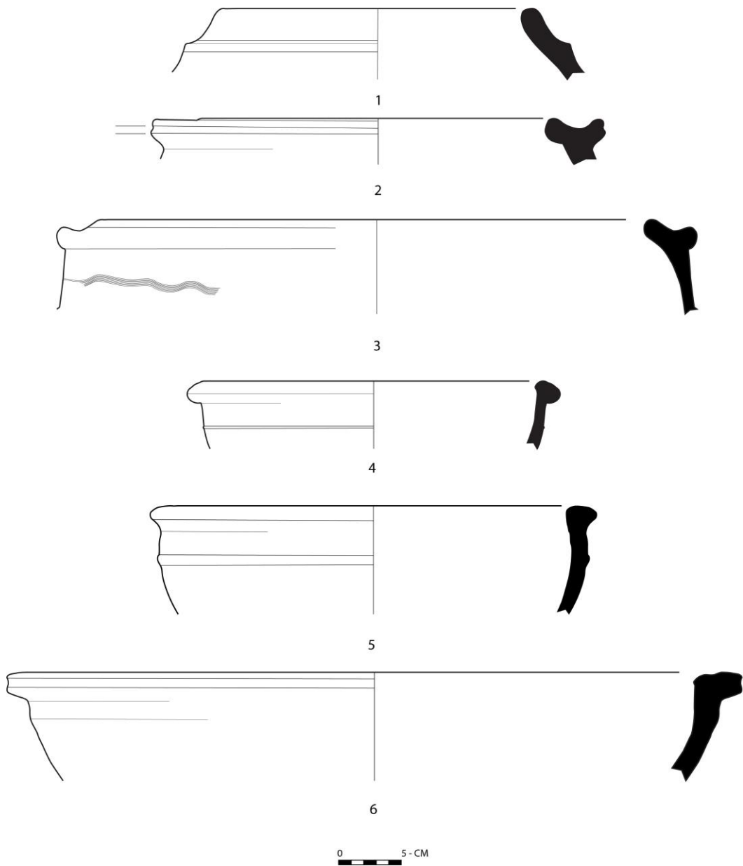
هنيلکاري (29)- هنيلکاري گلنپنهى هملبژير دراو له گردى روستهم، لنيوى گوزهى رووه و ناوهوه (3-1) و لنيوى قاپى قوولى رووه و دهرموه (5-4) و لنيوى تهشتى رووه و دهرموه (6)- (وينهکيشانى: H.B. Potts) و (هنيلکاري: تويژهر).
