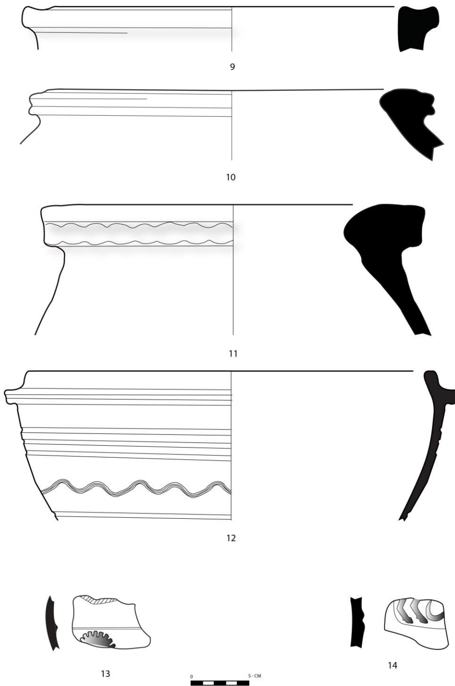
هیلکاری ژماره (2): نمونه‌ی گلینه‌ی هلبیزیردر او له گردی فلرخ، لیوی گوزه‌ی کونگاکردن (9، 11)، لیوی کووپه کهندوو (10) و لیوی قاپی قوول (12)، و پارچه گوزه (13-14)، : لیوی ریک (9) و لیوی رووه و ناوهه (10-12) - (هیلکاری: توئژهر).
