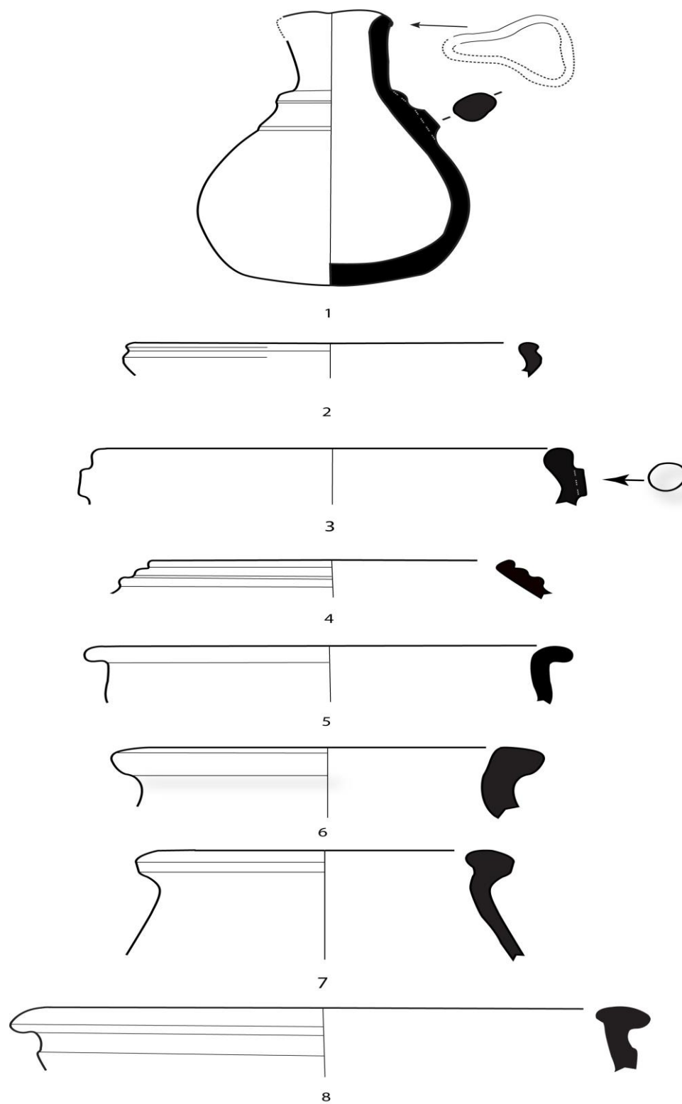
هیلکاری ژماره (1): نمونهی گلینهی هیلبیزیردراو له گردی قلرخ، لئیوی سوراحی (1)، قاپ (3-2)، گوزه (8-4): لئیوی پرووه ودمرموه (6,1) و لئیوی پرووه وناوموه (7, 4-2) و لئیوی رینک (8,5)-(هیلکاری: توئزهر).
