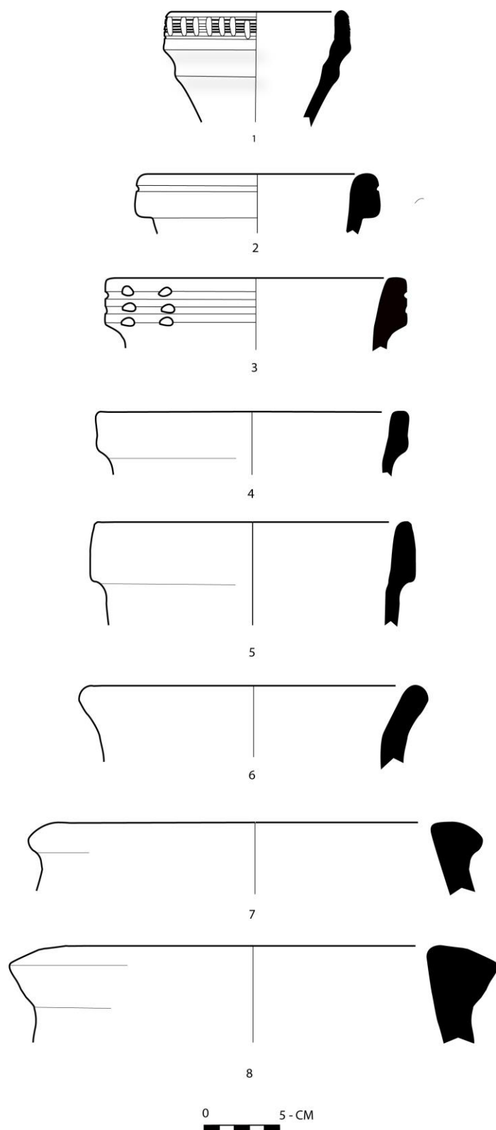
هیلکاری (15)- هیلکاری گلینه‌ی هلبیزیردر او له قه‌لای بازیان، لیوی کسموله (1) و نهمفور (2-5) و گوزه (6-8): لیوی پرووه و دهرهوه (6,1) و ریک (2-5) و پرووه و ناوهوه (7-8)- (هیلکاری: توئژمر).
