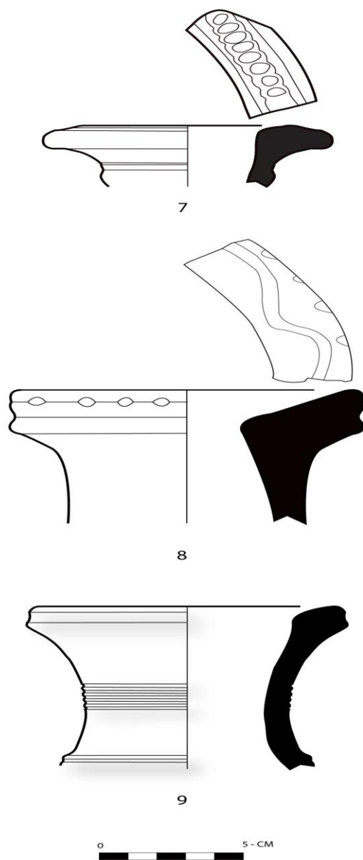
هیلکاری ژماره (5): نمونهی گلینهی هلبزیردر او له گردی کاژاو، لیوی گوزه: (7,9) لیوی رووه و دهر موه و (8) لیوی رووه و ناو موه (هیلکاری: توئزهر).
