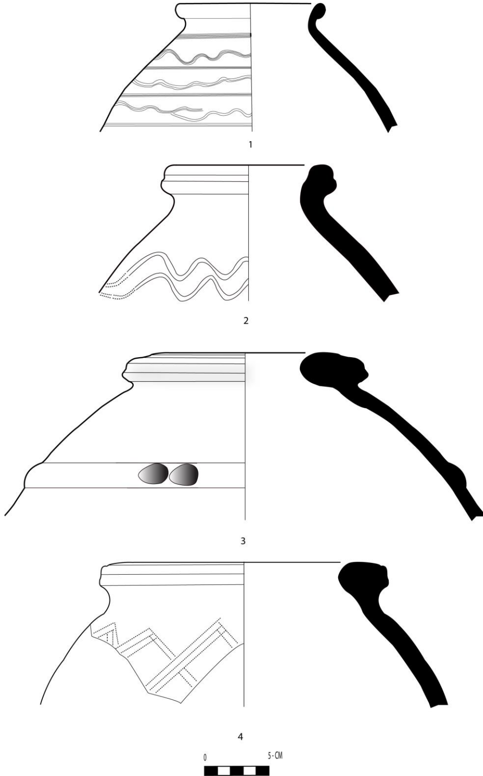
هیلکاری ژماره (3): نمونه‌ی گلینه‌ی هلبژیردر او له گردی کاژاو، لئیوی گوزه‌ی کوگاگردن (1-4، 2) و کووپه کهندوو (3)، : لئیوی رووه وده‌روه (1-2) و لئیوی رووه وناوه‌وه (3-4)- (هیلکاری: توپژهر).
