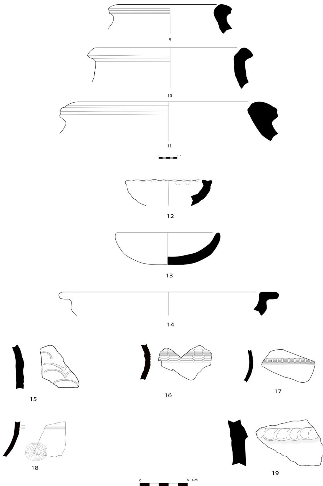
هیلکاری (16)- هیلکاری گنبنه می هملیژیر در او له قه لای بازیان، لیوی گوزه (9-10) و کوپه کمندو (11) و قاپ (12-14) و لاشه (15-19): لیوی پرووه و ناوموه (9,11) و پرووه و دهرموه (10,12,14)- (هیلکاری: توئژهر).
