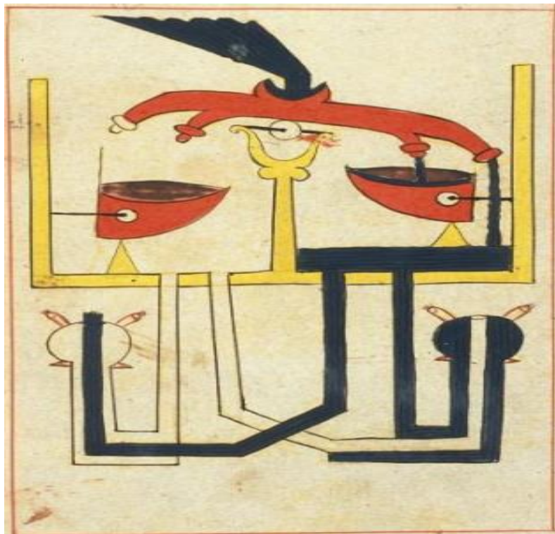
وینه ی ژماره (۶۵) (نافوردهی دوو لایی شیوه تهرازوو) وه ره قه ی ژماره (۱۰۴) له ده ستنوسی ژماره یه ک
