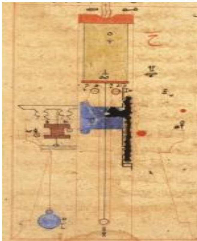
وينه ي ژماره (٣٢) (كاتزميرى نوسهر) وه ره قه ي ژماره (٥٨) له دهستنووسى ژماره يهك
