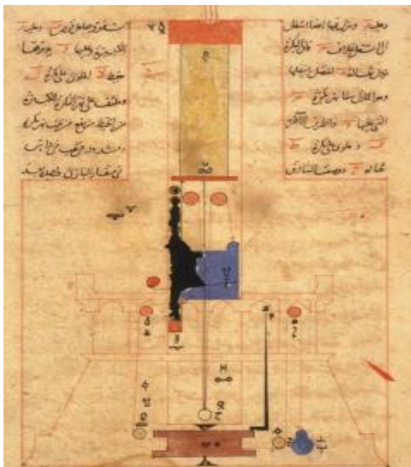
وینه‌ی ژماره‌(۳۴) (کاتژمی‌ری ده‌رگا) وه‌ره‌قه‌ی ژماره‌(۶۱) له ده‌ست‌نوس‌ی ژماره‌ یه‌ک
