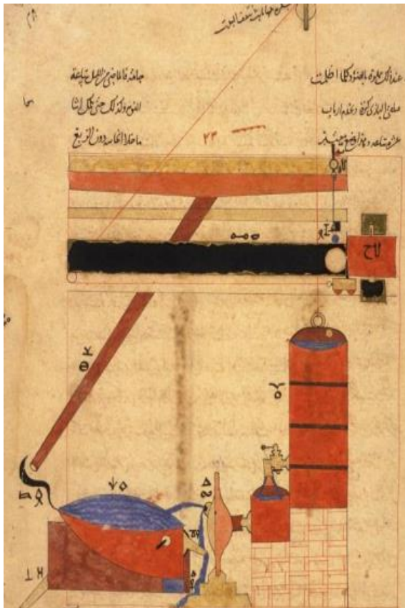
ويتهى ژماره (۲۰) به شيك له (کاتژميرى ته پل ليده رکان) و يتهى ژماره (۲۱) به شى ناوه وى کاتژميره که وه ره قهى ژماره (۲۴) له ده ستنوسى ژماره يه ک و يتهى ژماره (۲۸) له ده ستنوسى ژماره يه ک
