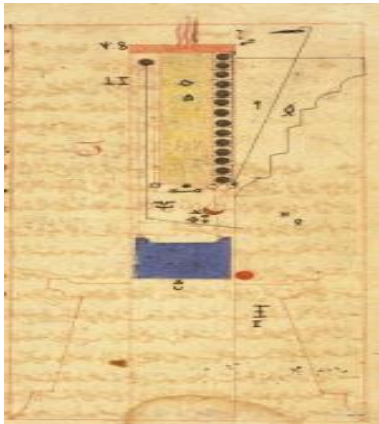
وینە ی ژمارە (۳۱) (کاتژمیری شمشیر) وەر قە ی ژمارە (۵۶) لە دەستتوسی ژمارە یەک
