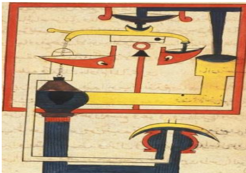
وینەى ژمارە ۶۹) نافورەى شىوھ چوارگۆشە وەرەقەى ژمارە ۱۱۲) لە دەستنووسى ژمارە يەك
