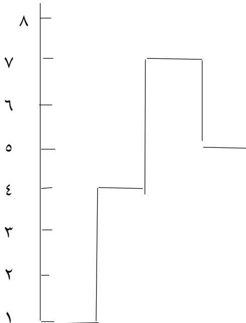
نه خشه ي (1) دابه شكردى برگه يى بو وشه ي (plaire)، هه ر به رزييه ك برگه يه كه
