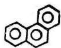
فینانترین (۱)
