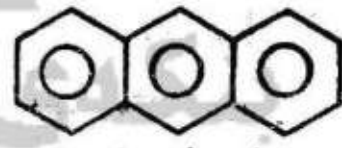
نه نتراسین (۲)
