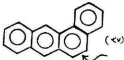
2,11-بهنزنه فلورین (۲۷)
