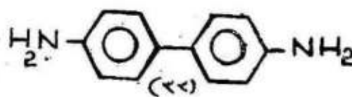
بە نزیدین
