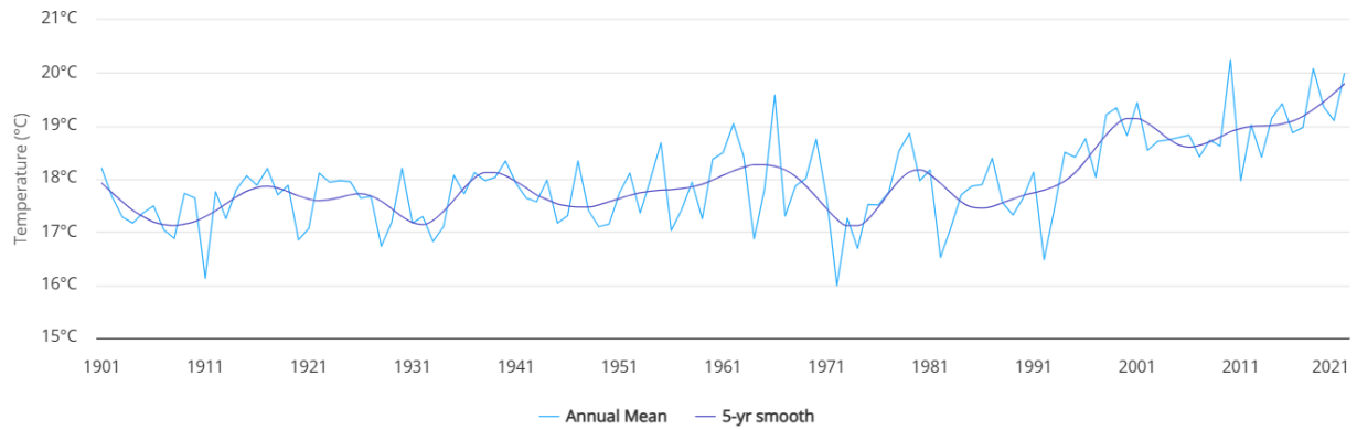
وینہی ۴: تیکرای پلهی گهرمی سالانهی چاودیرکراو له سلیمانی و هه نه بجه (۱۹۰۱-۲۰۲۱)
