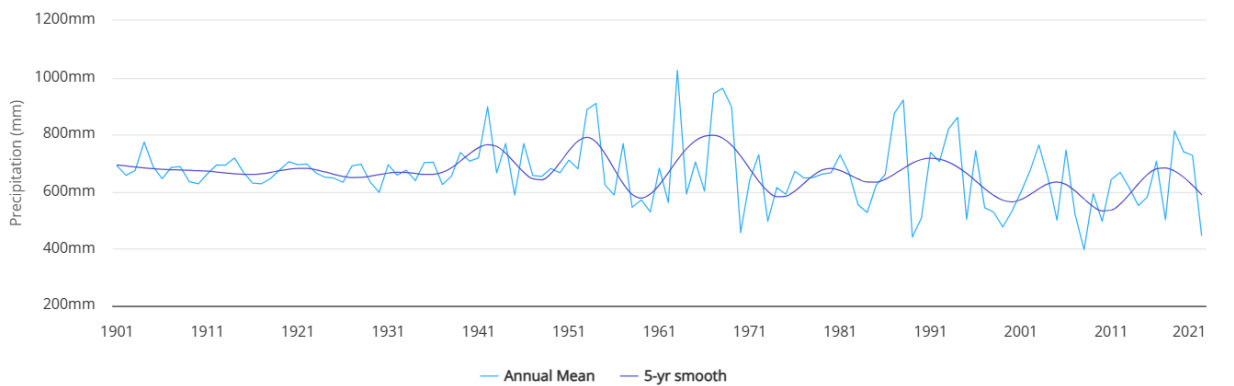
وینە ۱۱: تیکرای بارانبارینی سالانه که له دهۆک بهدی کراوه (۱۹۰۱-۲۰۲۱)
