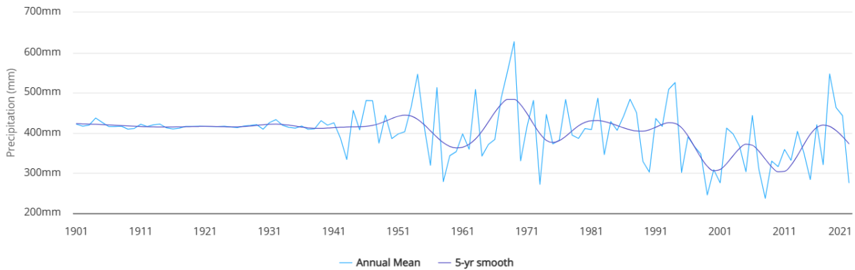
وینە ۱۰: تیکرای بارانبارینی سالانه که له سلیمانی و ههلهبجه بهدی کراوه (۱۹۰۱-۲۰۲۱)
