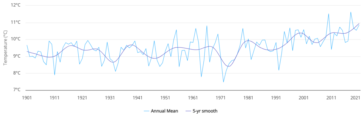
وینہی ۸: تیکرای که مترین پله کانی گهرما که سالانه له دهوک بهدی کراوه (۱۹۰۱-۲۰۲۱)
