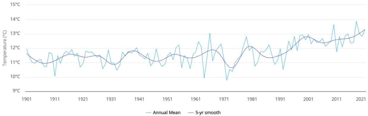
وینہی ۷: تیکرای که مترین پلهی گهرما که سالانه له سلیمانی و ههلهبجه بهدی کراوه (۱۹۰۱-۲۰۲۱)
