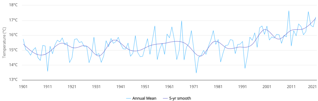
وینہی ۵: تیکرای مامناوهندی پلهی گهرمی سالانهی چاودیرکراو له دهوک (۱۹۰۱-۲۰۲۱)
