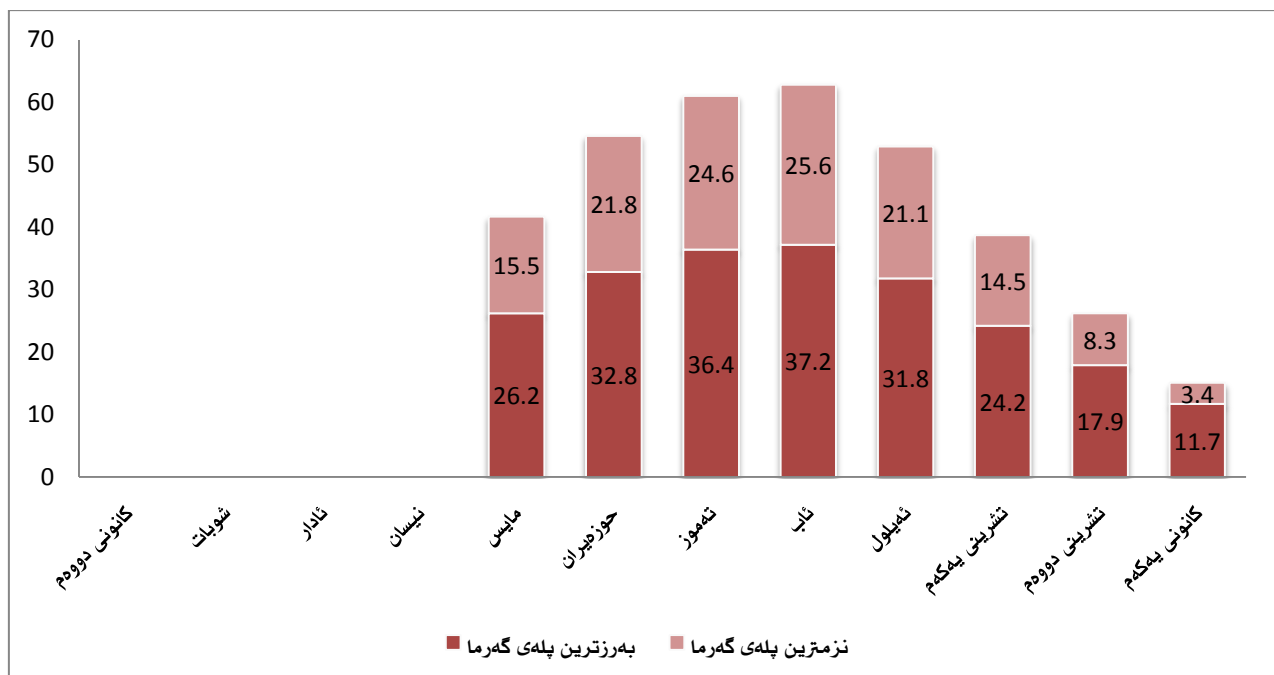
پلەى گەرما بۇ مانگەكانى سالى 2008 لە پىرام (سەلاھەدىن)
