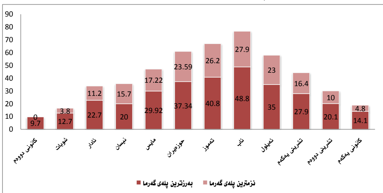
پلەى گەرما بۇ مانگەكانى سالى 2008 لە پارىزگاي دەۋك
