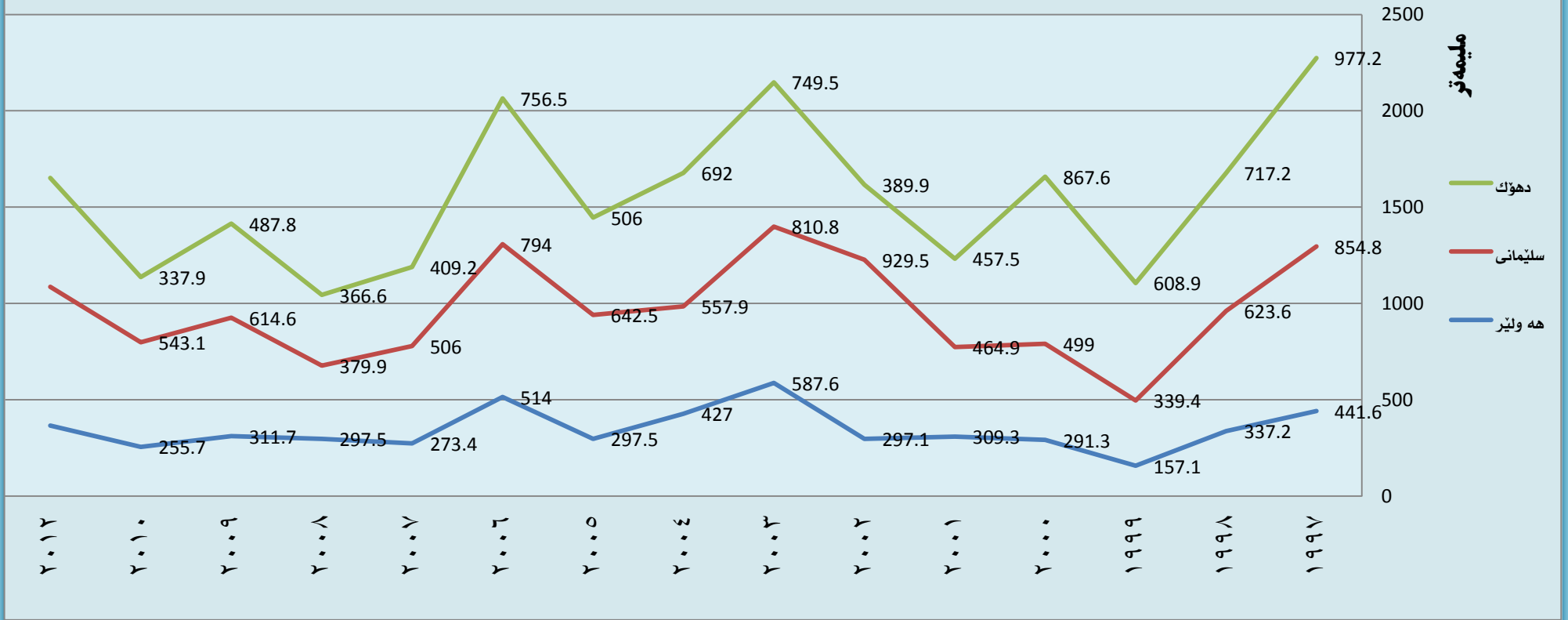
برې باران بارين له پاريزگانى ههريمي كوردستان به (مليمهتر) بۆ سالانى ۱۹۹۷ تا ۲۰۱۲
