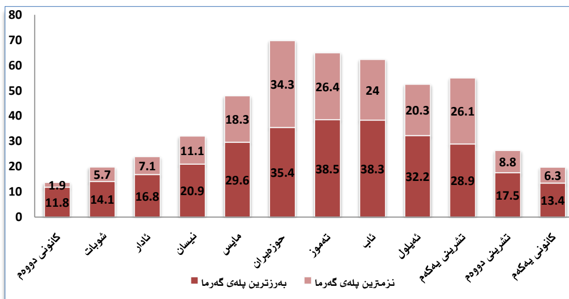
پله‌ی گهرما بۆ مانگه‌کانی سالی 2009 له پارێزگای سلێمانی
