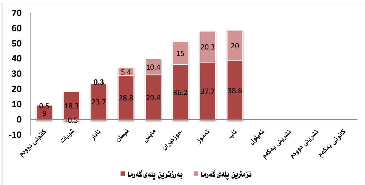
پلەى گەرما بۆ مانگەکانى سالى 2013 لە پیرمام
