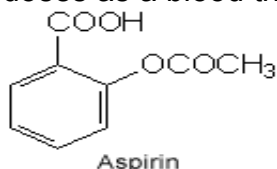
Aspirin
